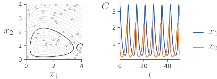
FIGURE 2.7 – Modèle de Lotka-Volterra à deux populations. Gauche : Champ vectoriel de la dynamique pour c_1 = 1.0, c_2 = -1.0, W_{12} = 1.2, W_{21} = -0.8 . On voit que le point d'équilibre est bien un centre pour la dynamique non linéaire dans ce cas et la courbe C désigne un des cycles limites associés au point d'équilibre. Droite : Trajectoires des populations x_1 et x_2 sur le cycle limite C .
