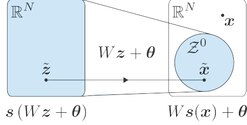
FIGURE 3.2 – Relation entre les deux formes de dynamiques de RNN. La partie de gauche représente le système de l'Éq.(3.158), tandis que la partie de droite représente le système de l'Éq. (3.148). La transformation affine Wz + \theta envoie l'entièreté du système de gauche vers le sous-ensemble \mathcal{Z}^0 dans le système de droite. Tout x \notin \mathcal{Z}^0 ne possède donc pas d'équivalent dans le système de gauche.
