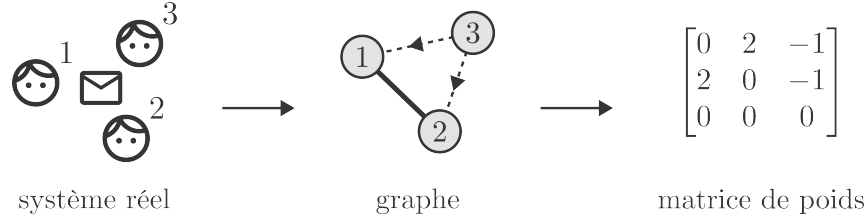
FIGURE 2.2 – Représentation par un graphe d’un réseau d’échange de messages. Les trois personnes correspondent aux N = 3 sommets du graphe et les arcs représentent les messages envoyés. Le poids correspond au nombre quotidien de messages. Les messages encourageants sont de signe positif et les messages haineux sont de signe négatif.
