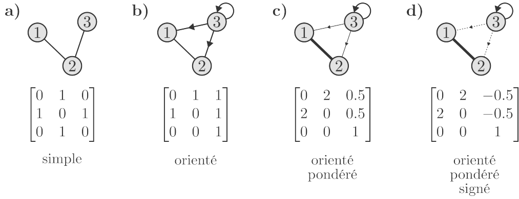
FIGURE 2.1 – Différents types de graphe et leur matrice d’adjacence/de poids associée. Les sommets sont représentés par des cercles indicés, tandis que les arêtes/arcs sont représentés par des traits. a) Un graphe simple possède une matrice d’adjacence symétrique. b) Un graphe orienté possède une matrice d’adjacence qui n’est pas forcément symétrique. De plus, ce graphe possède la boucle (3,3). c) Un graphe orienté et pondéré possède une matrice de poids avec des éléments non négatifs. Sur le dessin, les poids sont représentés par l’épaisseur du trait. d) Un graphe orienté, pondéré et signé possède une matrice de poids générale. Les arcs de signe positif sont dessinés avec un trait plein et les arcs négatifs sont pointillés.
