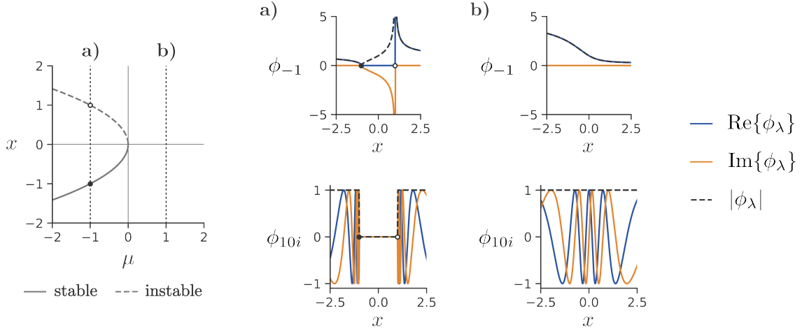
FIGURE 1.4 – Fonctions propres de la forme normale de bifurcation noeud-selle. À gauche : Diagramme de la bifurcation noeud-selle. Les courbes pleine et pointillée désignent respectivement la positions du point d'équilibre stable et instable. À droite : Fonctions propres du GOK de valeur propre -1 (haut) et 10i (bas) pour les paramètres a) \mu = -1 et b) \mu = 1 . En haut, on observe bien que les zéros et les singularités de la fonction propre concordent avec les points d'équilibre du diagramme de bifurcation, tandis qu'en bas, la norme est conservée sur chaque ensemble invariant (propriétés attendues par le Lem. 27).
