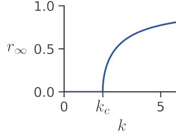
FIGURE 2.3 – Paramètre d'ordre de Kuramoto en fonction du couplage. Diagramme du paramètre d'ordre r_\infty dans la limite t \rightarrow \infty et N \rightarrow \infty pour la distribution de Cauchy G(\omega) = (\pi(\omega^2 + 1))^{-1} . Dans ce cas, la distribution est centrée autour de \mu = 0 . Comme G(0) = 1/\pi , l'Éq. (2.10) donne un couplage critique de k_c = 2 .
