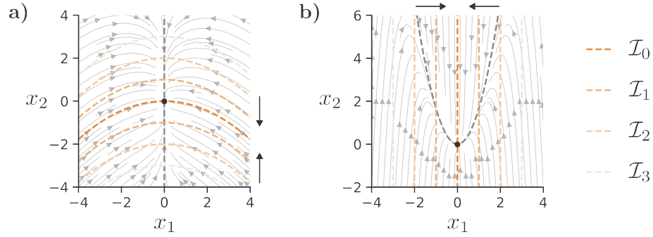
FIGURE 1.3 – Exemple simple d'isostables. a) Pour \nu = -0.2 et \mu = -1 , les isostables sont données par les courbes de niveau de |\phi_2| . b) Pour \nu = -1 et \mu = -0.2 , les isostables sont plutôt les courbes de niveau de |\phi_1| . Dans les deux cas, les flèches dénotent la convergence exponentielle des trajectoires vers l'isostable \mathcal{I}_0 et la courbe grise pointillée désigne l'ensemble des zéros de l'autre fonction propre.
