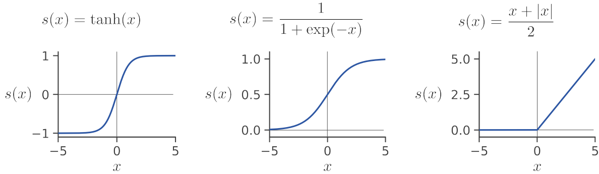
FIGURE 2.4 – Exemples courants de fonction d’activation. Les fonctions de gauche (tangente hyperbolique) et du centre (sigmoïde) sont analytiques, tandis que la fonction de droite ( Rectified Linear Unit ou ReLU) n’est pas continûment dérivable.
