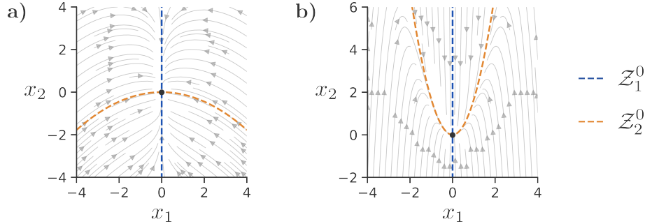
FIGURE 1.2 – Ensembles des zéros des fonctions propres pour a) \nu = -0.2 , \mu = -1 et b) \nu = -1 , \mu = -0.2 . Les courbes bleue et orange sont respectivement les ensembles des zéros de \phi_1 et de \phi_2 et sont des ensembles invariants. Les deux courbes se croisent à l'origine, où se trouve un point d'équilibre globalement stable.
