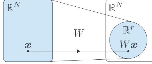
FIGURE 2.8 – Représentation conceptuelle du rang d’une matrice. La matrice W de taille N \times N et de rang r est associée à une transformation linéaire envoyant les vecteurs de \mathbb{R}^N vers un sous-espace de \mathbb{R}^N de dimension r .
