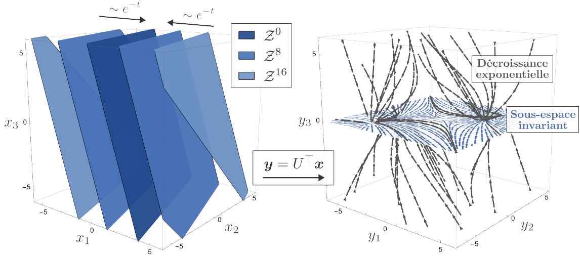
FIGURE 3.1 – RNN avec une fonction propre linéaire. Gauche : Les courbes de niveau \mathcal{Z}^C de l'Éq. (3.157), montrées ici pour C = 8 et C = 16 , sont des quantités analogues aux isostables pour le sous-espace invariant attractif \mathcal{Z}^0 . Droite : Champ vectoriel de la dynamique en \mathbf{y} . Sous le changement de variables \mathbf{y} = U^\top \mathbf{x} , le sous-espace invariant est défini par y_3 = 0 . Les trajectoires convergent vers ce sous-espace en \sim \exp(-t) .
