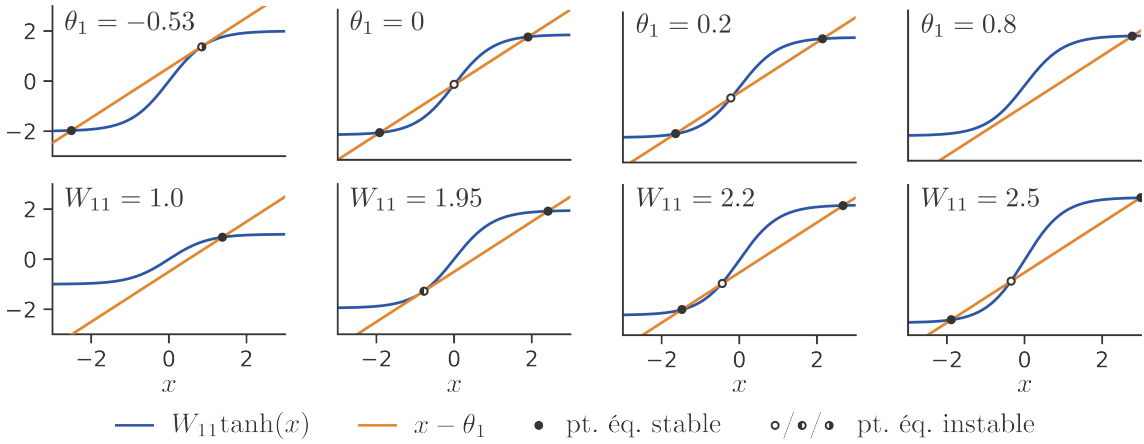
FIGURE 2.5 – Points d'équilibre du neurone en auto-interaction. Haut : Membres gauche et droit de l'Éq. (2.24) pour un poids W_{11} = 2 avec différentes valeurs de \theta_1 . Bas : Membres gauche et droit de l'Éq. (2.24) pour \theta_1 = 0.5 avec différentes valeurs de W_{11} . Dans les deux cas, on observe que le système possède 1, 2 ou 3 points d'équilibre. Pour les points d'équilibre instables, les côtés pleins désignent un côté où les trajectoires convergent vers le point d'équilibre (parfois appelés points d'équilibre semi-stables , de tels points d'équilibre sont instables selon la Déf. 3).
