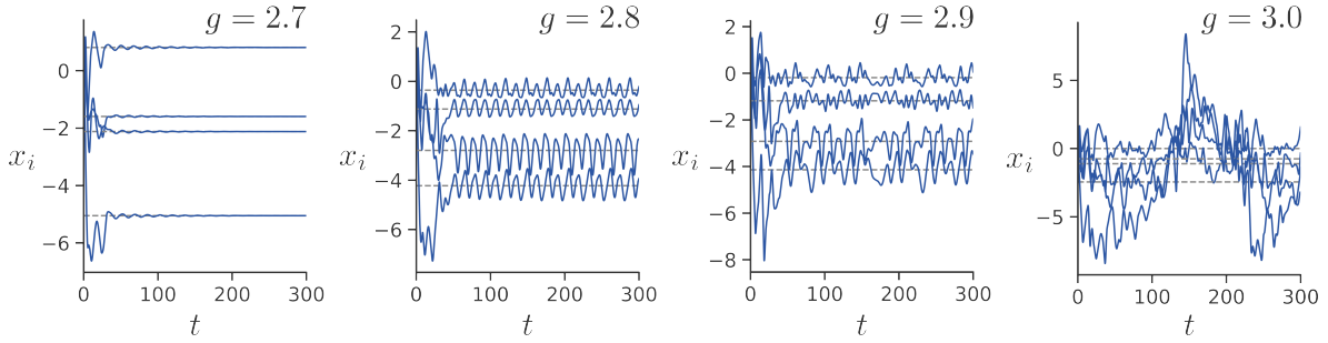
FIGURE 2.9 – Régimes d’activité d’un RNN aléatoire avec perturbation de rang 1. Les trajectoires montrées sont celles d’un échantillon de 4 neurones pour un système avec N = 100 . La matrice Q = \mathbf{m}\mathbf{n}^\top/N de rang 1 est construite à partir de deux vecteurs \mathbf{m}, \mathbf{n} tirés d’une distribution normale centrée à 1.5 et de variance 1. Dans la réalisation montrée ici, \mathbf{m}^\top \mathbf{n}/N \approx 2.74 (cette quantité est la force de la structure ou structure strength de [60]). La partie aléatoire \chi est tirée d’une distribution normale centrée à 0 de variance 1/N . Pour g = 2.7 , l’activité converge vers un point d’équilibre. Pour g = 2.8 , le système semble plutôt converger vers un cycle limite. Pour g = 2.9 , on observe le régime le plus intéressant, car le système possède un comportement chaotique où l’activité reste près d’une valeur moyenne distincte pour chaque neurone. Finalement, pour g = 3.0 , le comportement chaotique domine sur le comportement structuré et les trajectoires s’éloignent davantage des valeurs moyennes. Dans chaque cas, les lignes grises pointillées sont les valeurs moyennes des trajectoires sur t \in [30, 300] .
