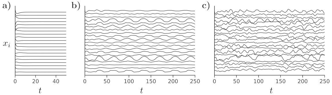
FIGURE 2.6 – Séries temporelles d'un RNN en régimes chaotique et non chaotique. Le RNN comporte N = 100 neurones sur un graphe aléatoire de variance w^2/N . Les séries temporelles d'un échantillon de 20 neurones sont montrées ici. Dans tous les cas, la constante g est fixée à 1. a) Pour w = 0.8 , le paramètre de gain G est plus petit que 1 et le système converge vers un point d'équilibre. b) Pour w = 1.5 , le paramètre de gain G est entre 1 et 2 et le système converge vers un cycle limite. c) Pour w = 2.5 , le paramètre de gain est plus élevé que 2 et on observe un comportement chaotique.
