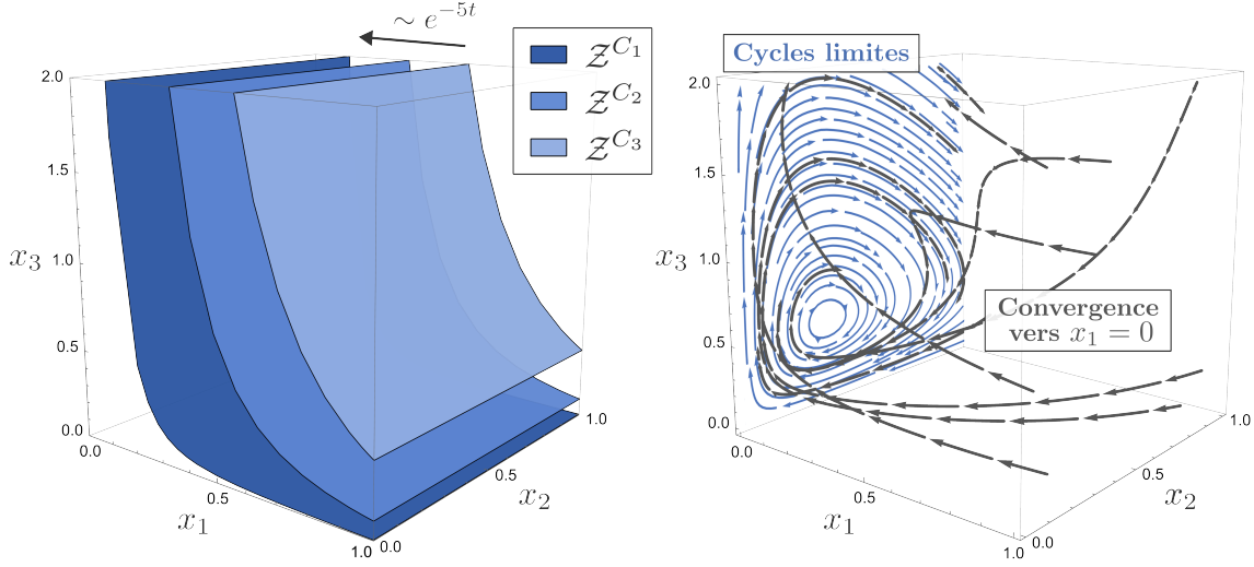
FIGURE 3.3 – Lotka-Volterra avec une fonction propre monomiale. Gauche : Les ensembles de niveau de |\phi_3| pour C_1 = 0.005 , C_2 = 0.1 et C_3 = 0.4 montrent la convergence vers x_1 = 0 ou x_3 = 0 . Droite : Numériquement, les trajectoires montrent une convergence vers x_1 = 0 . Sur ce sous-espace, on observe les cycles limites du système de Lotka-Volterra à deux populations défini par x_2 et x_3 .
