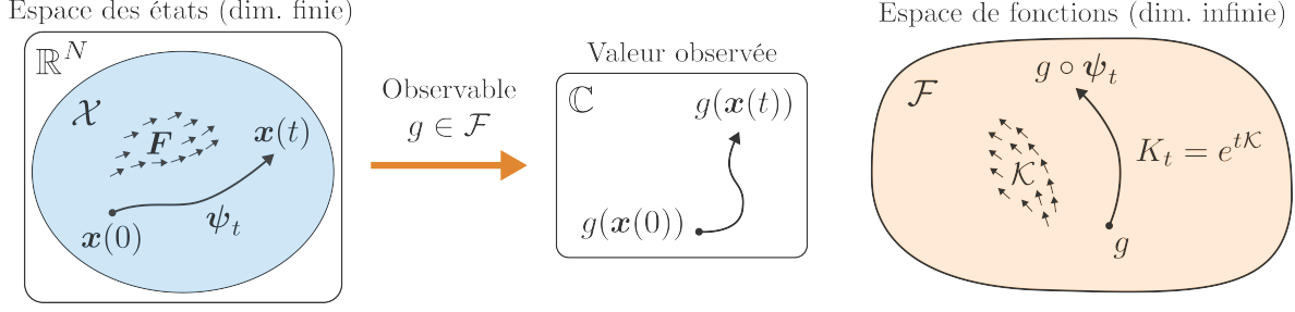
FIGURE 1.1 – Représentation schématique de l’opérateur de Koopman et de son générateur. Dans l’espace des états \mathcal{X} , qui est de dimension finie N , la dynamique des états est régie par un champ vectoriel (possiblement non linéaire) \mathbf{F} qui génère le flot \psi_t . Dans l’espace de fonctions \mathcal{F} , qui est de dimension infinie, la dynamique des observables est linéaire et est régie par l’opérateur de Koopman K_t et son générateur \mathcal{K} . Les deux descriptions permettent de décrire l’évolution dans le temps de la valeur observée g(\mathbf{x}(t)) .
